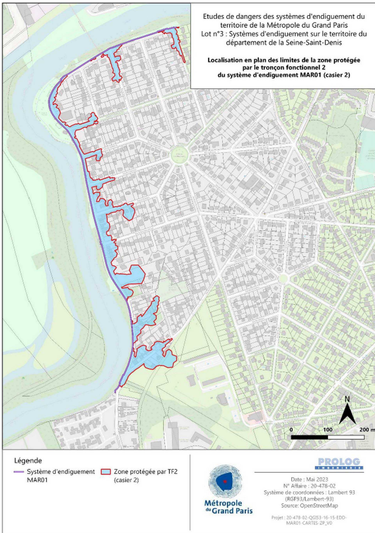
Tronçon fonctionnel n°2
