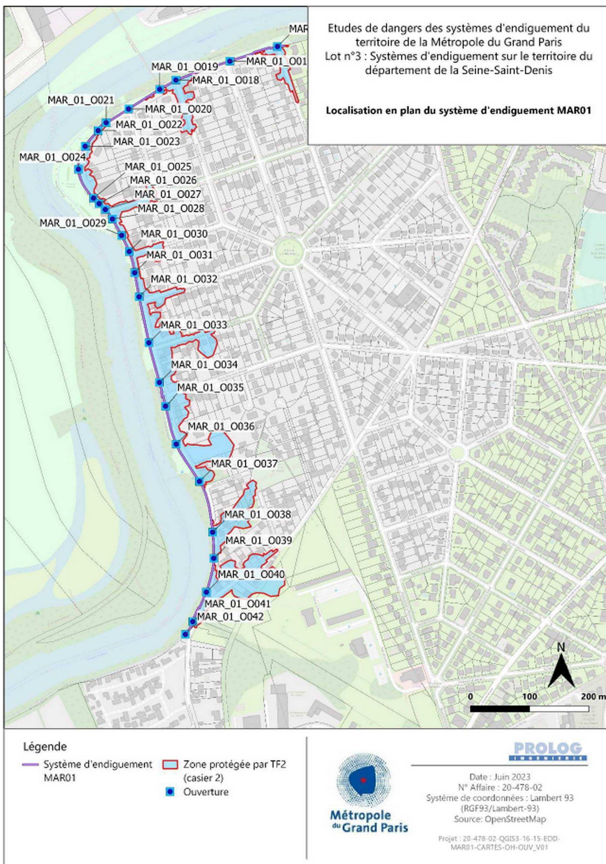
Ouvertures batardables sur le tronçon fonctionnel n°2
